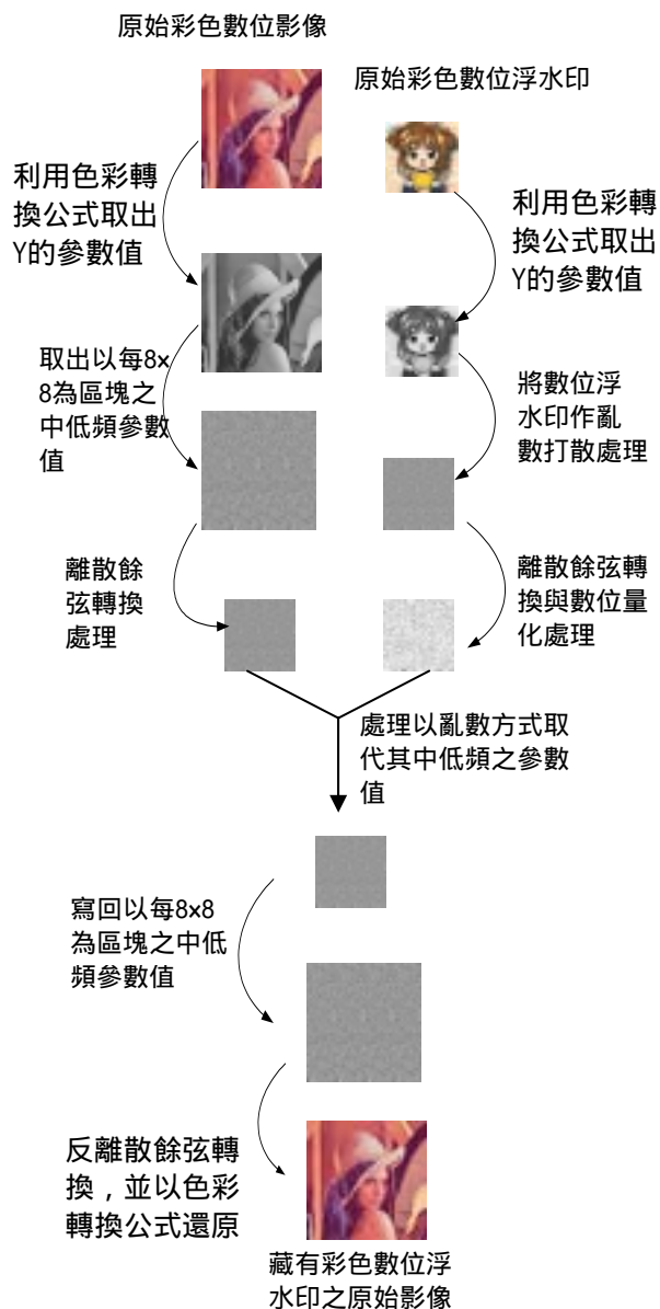
【圖 5】彩色數位浮水印藏入流程圖
