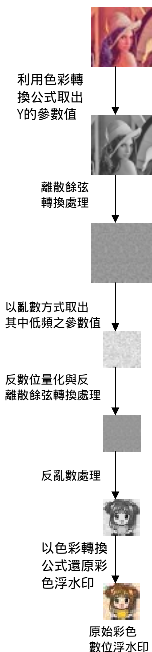
【圖 6】彩色數位浮水印取回流程圖
