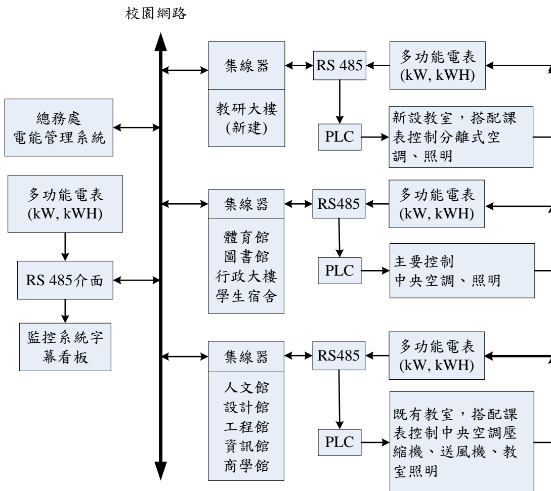
圖 2 網控電能管理系統基本架構
