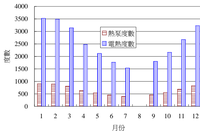
圖 10 不同月份平均日耗電量比較
