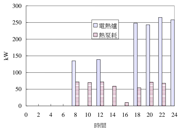
圖 9 每日加熱運轉時間及耗電功率曲線
