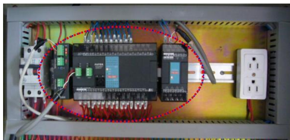
圖 3(b) PLC 外觀
