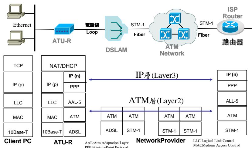
圖 2. ATM PVC-based 網路架構( ADSL )
