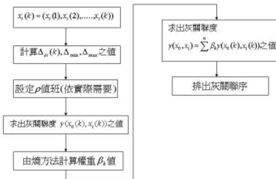
圖 4. 局部性灰關聯度作法流程圖(資料來源[5])
