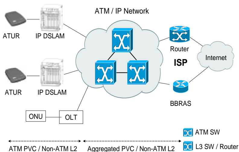
圖 3. 全 IP-based 網路架構( ADSL2 )
